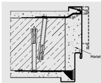
Prinzipskizze: Vorhandene, komplett in Massivwand ausge- mörtelte Stahlzarge
